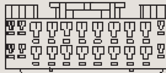
22ピン
