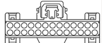
26ピン
