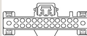
24ピン
